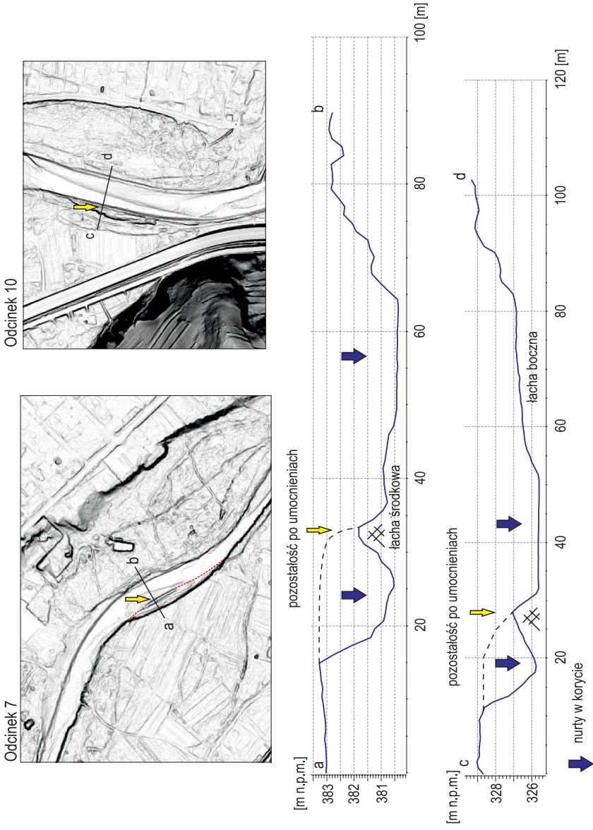
Ryc. 26. Przykład odcinków ze zniszczonymi umocnieniami – strefy poszerzania koryta Raby
