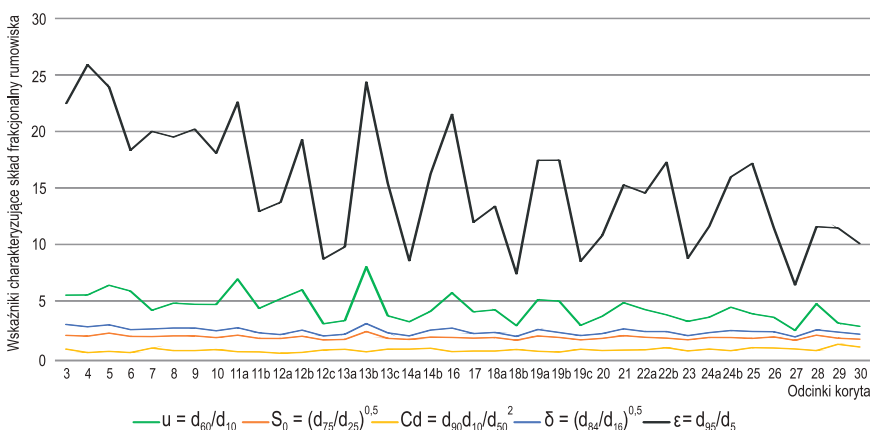
Ryc. 11. Wskaźniki charakteryzujące skład frakcjonalny rumowiska dla prób powierzchniowych
