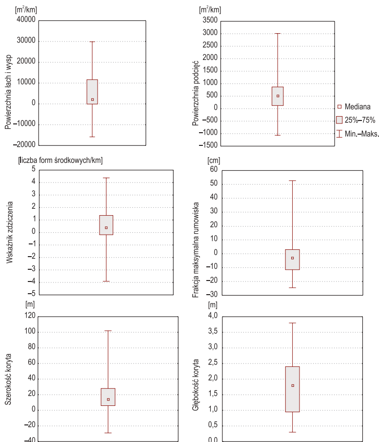
Ryc. 15. Wykres rozkładu empirycznego różnic cech struktury Raby w latach 1965–1976
